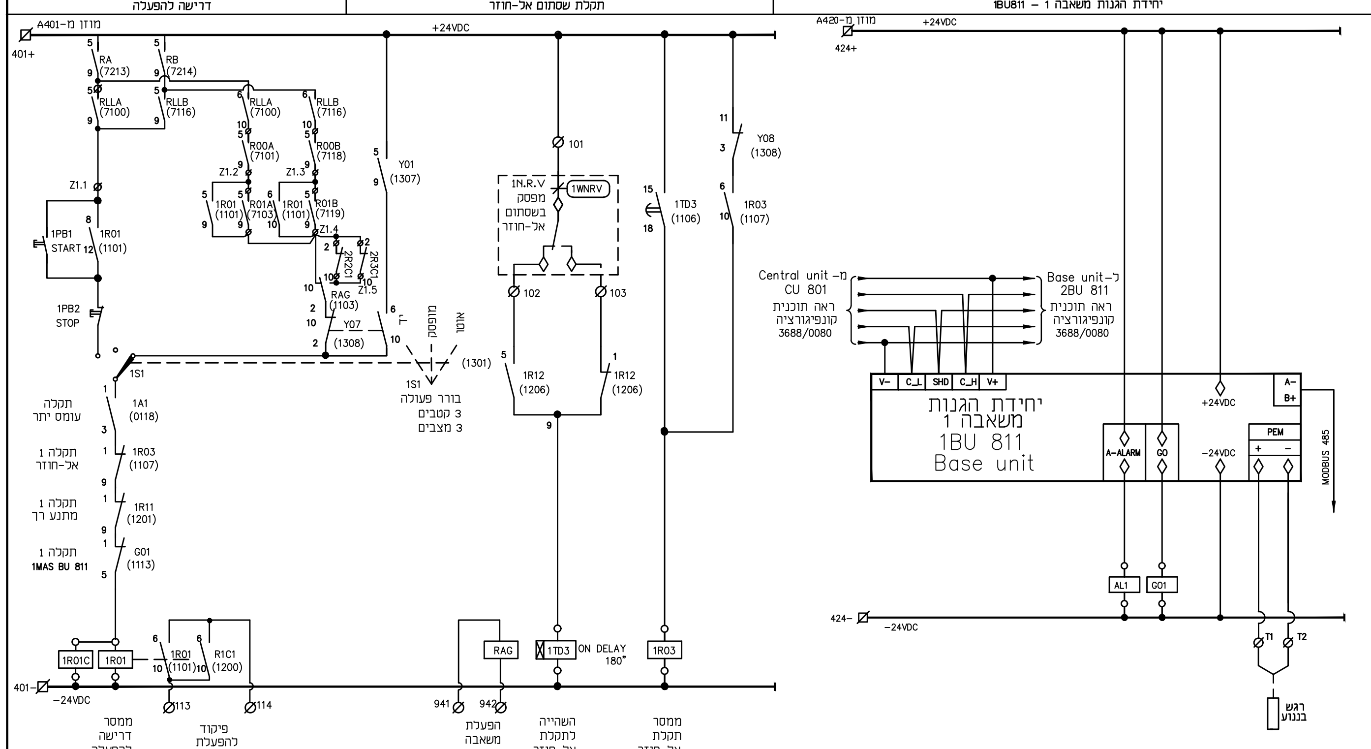
תא משאבה 1 הערה: טיפוי לשאר המשאבות בשינוי אינדקס - הקבלן יגיש לאישור סט תוכניות מלא!
